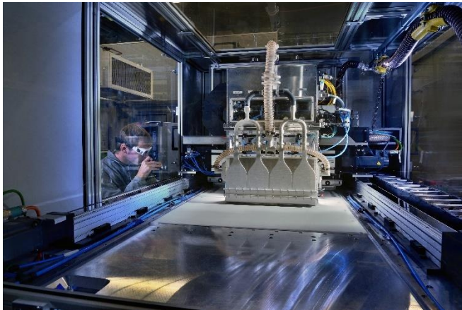
Bild 1: XXL on-the-Fly: Wie eine Gantry-Anlage mit dem laserbasierten Pulverbettverfahren (LPBF) große Bauteile aus Edelstahl herstellt, demonstrierte das Fraunhofer ILT auf dem AKL'22 beim 3D-Druck eines 300 mm hohen Rolls-Royce-Turbinenbauteil mit 650 mm Durchmesser.
