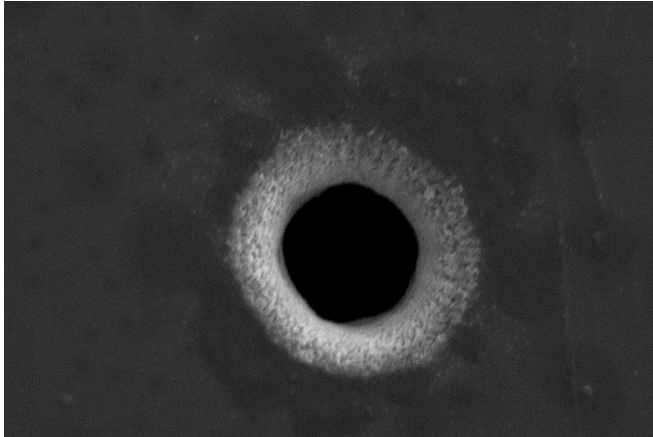
Bild 3: Mikrobohrung in einer Edelstahlfolie mit einem Austrittsdurchmesser von unter 10 Mikrometern. © Fraunhofer ILT, Aachen.
