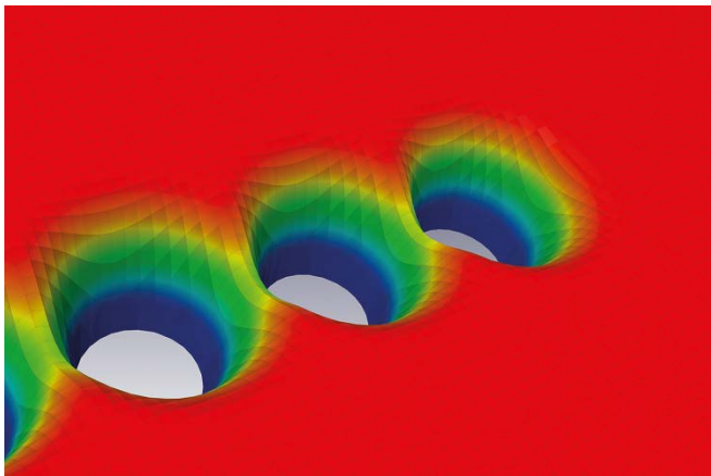
Bild 2: Simulation: Für den Bohrprozess werden die Bohrlochform und die Wärmebelastung berechnet und so die optimalen Laserparameter bestimmt. © Fraunhofer ILT, Aachen.
